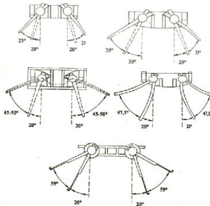
Рис. 98. Углы между крайними положениями рычага в машинах типа Марк III, Марк IIa (верхний ряд), Марк IIIb, усовершенствованном Марк IVa (средний ряд) и кейробаллисте (нижний рисунок)
